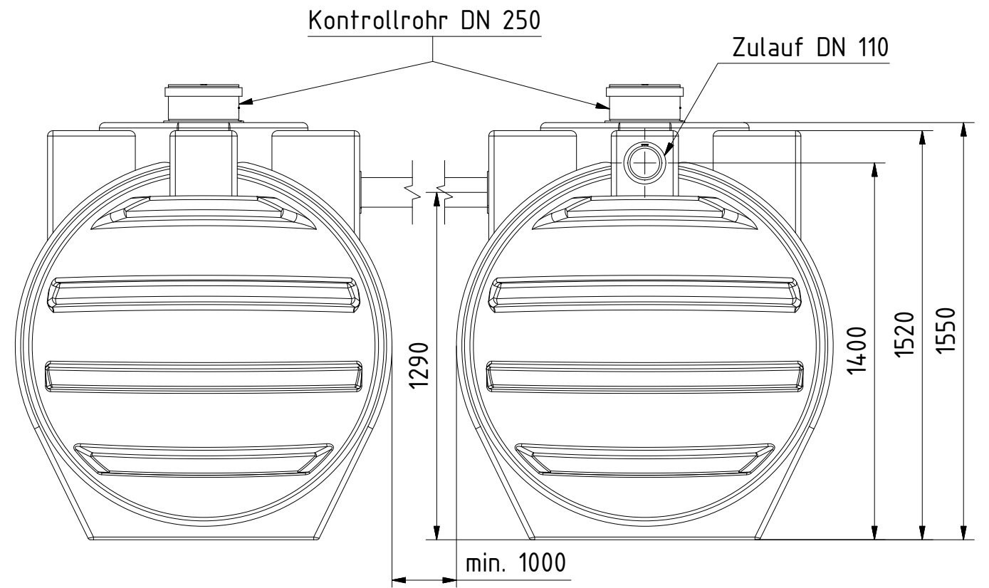
Frontansicht
